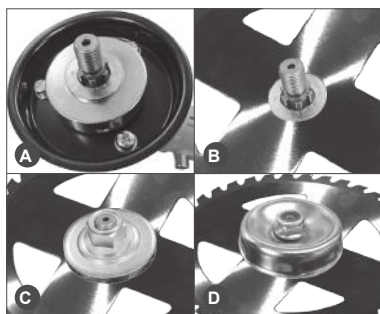
Рис. 5 Установка ножа
