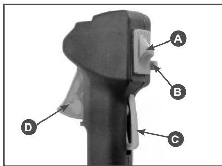
Рис.10 Расположение органов управления на рукоятке
