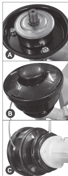
Рис. 6 Установка триммерной головки
